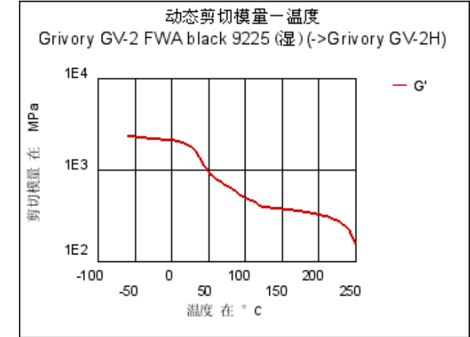
动态剪切模量 - 温度
